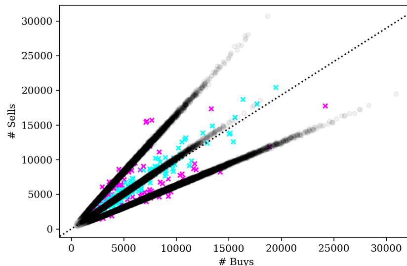
(d) BZH 2012
