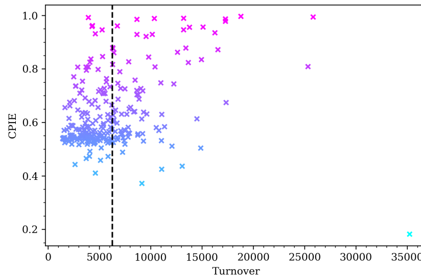
(d) TDSC 2012
