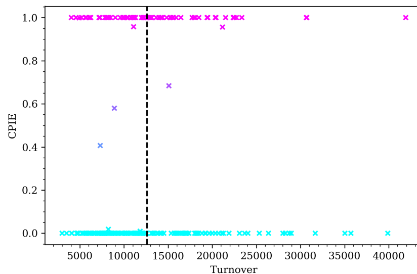
(d) BZH 2012
